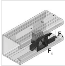
Stex 45 płytki montażowe MP-X
